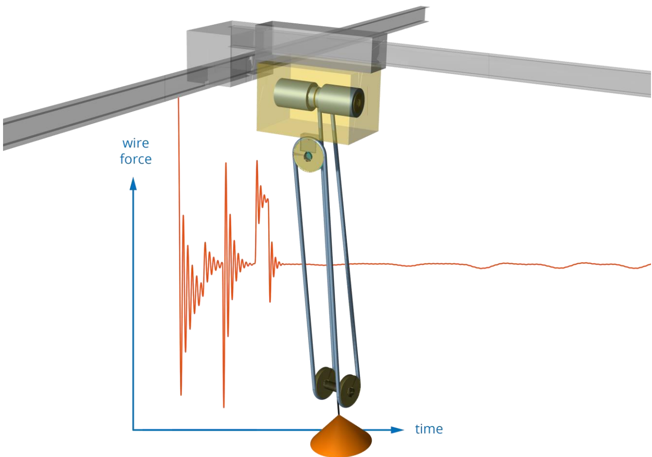
Image : Simulation en trois dimensions dans SimulationX 3.8 d'ESI : systèmes de l'entraînement par câbles et courroies de transmission.
